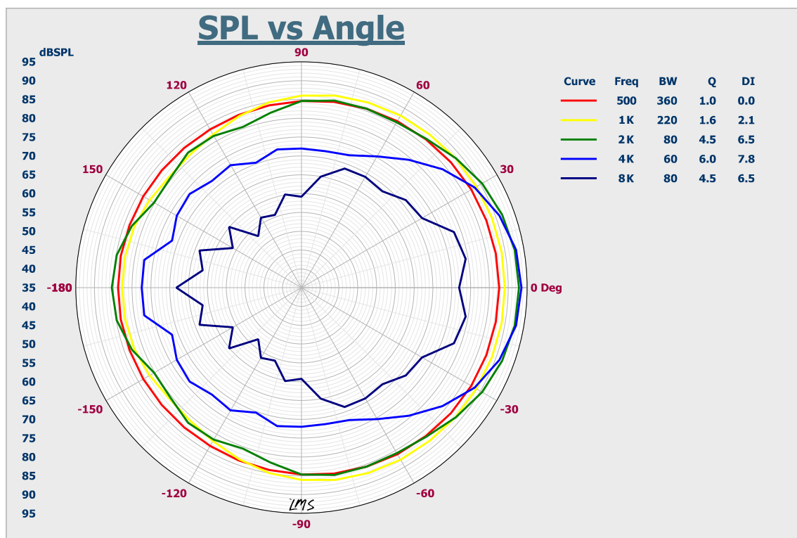
Круговая диаграмма направленности громкоговорителя LPA-10P
